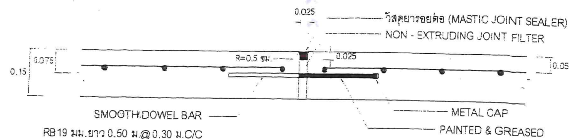
ขยายรอยต่อ EXPANSION JOINT
