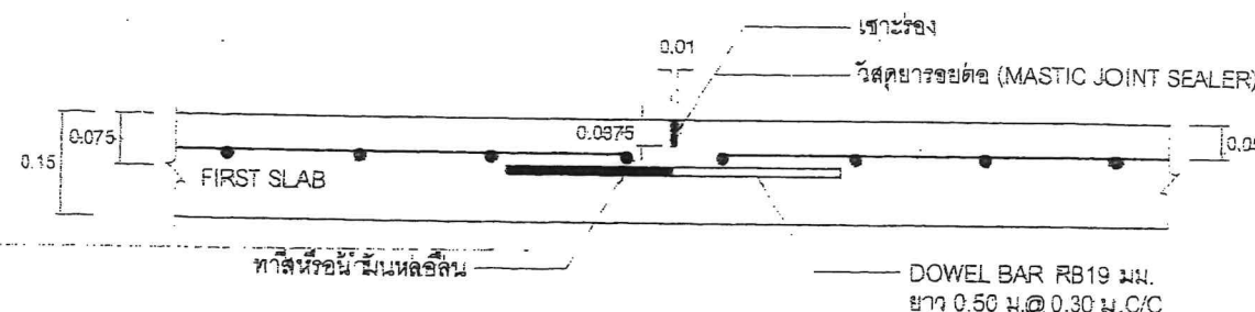
ขยายรอยต่อ CONSTRUCTION JOINT
